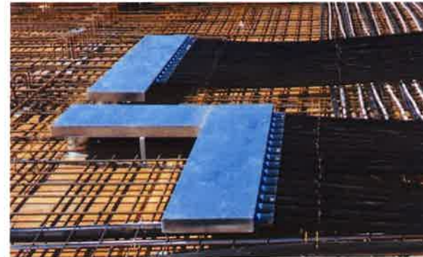
Distributeur de dalle sur mesure Eco-Confort SA Epaisseur 7 cm à l'axe de la dalle pour tubes diam. 47mm
